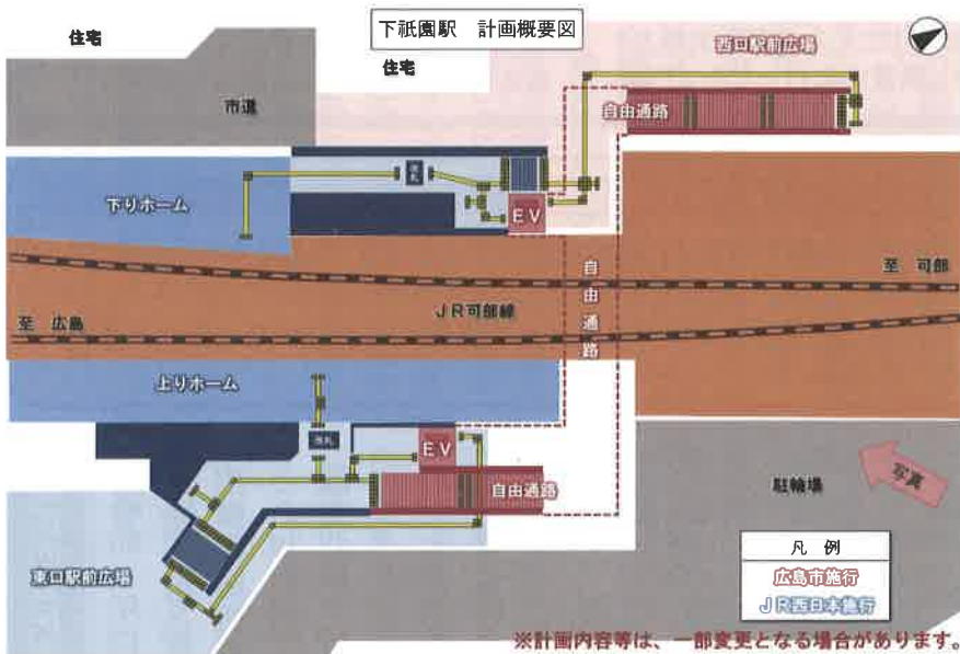
JR下祇園駅計画概要図 (広島市提供)
